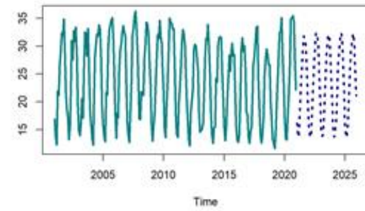
Forecasting of Vapour.Pressure till 2025
